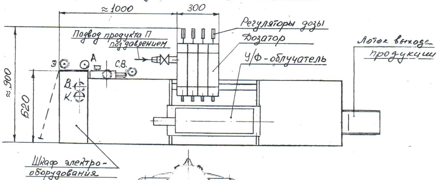
Рис. 1. Габаритные размеры и места подключения роликовочной автоматической линии мод. АЛБ 165
